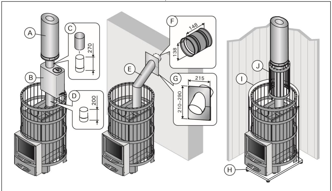
Figure 17. Accessories (all dimensions in millimeters) Abbildung 17. Zubehör (alle Abmessungen in Millimetern) oberen Anschlussöffnung. Wenn ein Schutzmantel
