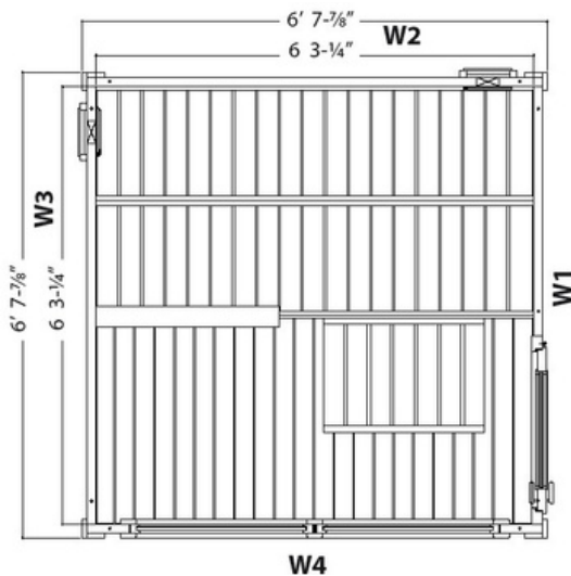
Sauna Floor Plan Right Hand:
